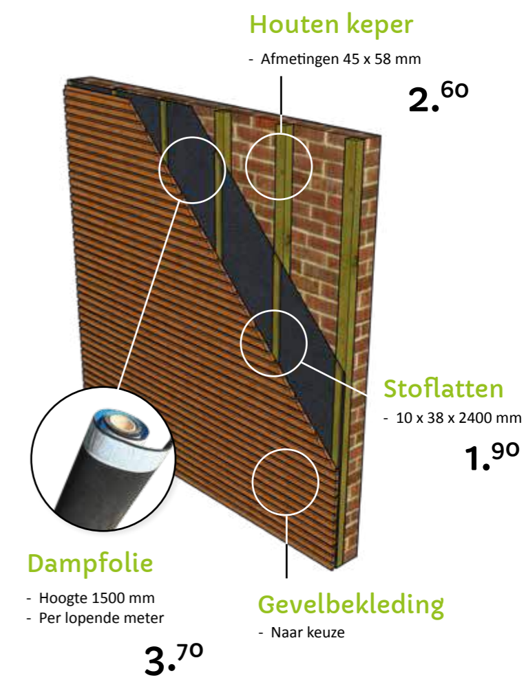
Gevelplank Thermowood line zie pag. 60
