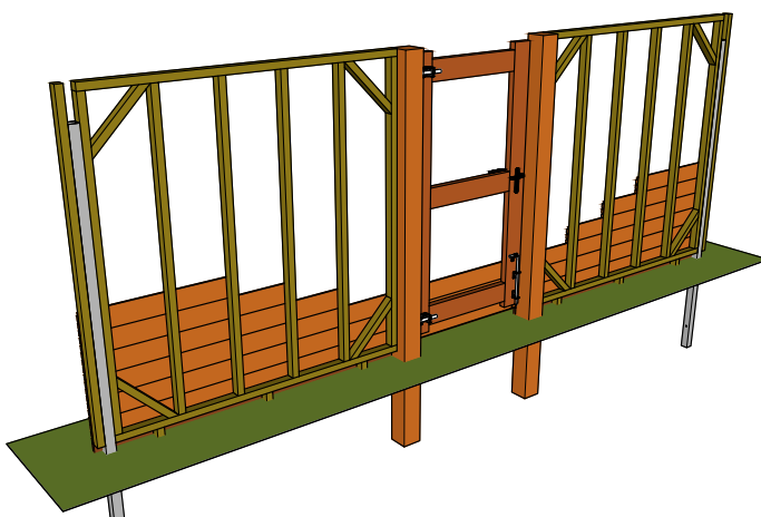
Achter aanzicht
